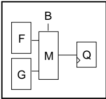
IOB—Base IO (2000, 3000, 4000, 5200)
