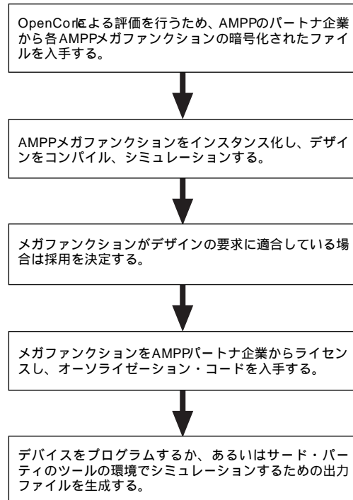
図 2 AMPP メガファンクションを評価するときのデザイン・フロー
