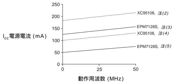
図2 MAX 7000SとXC9500の消費電力 注(1)
