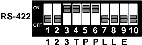
Figure 2 - RS-422
