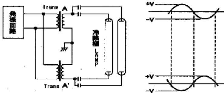
●图 4 정적냉음극용 Inverter
