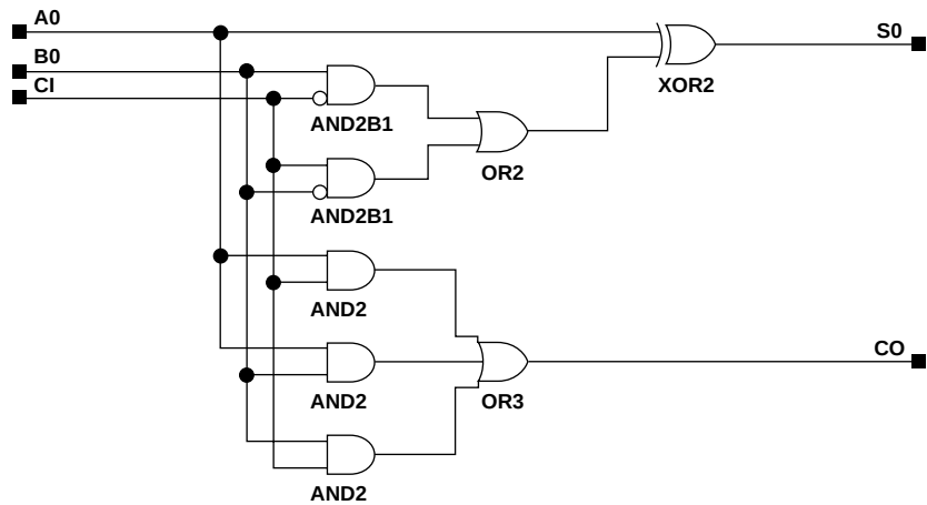
Figure 3-8 ADD1 Implementation XC9000
